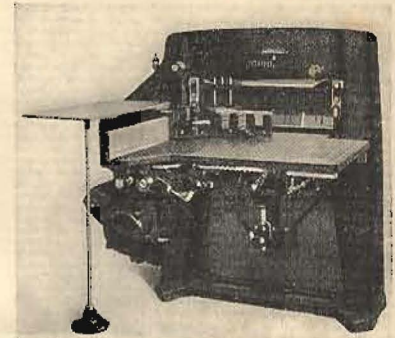
JOHNE Schnellteiler AK Schnittlänge 62 cm
