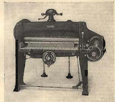
Schnellschneider IOHNE AS Schnittlängen 78 und 105 cm
